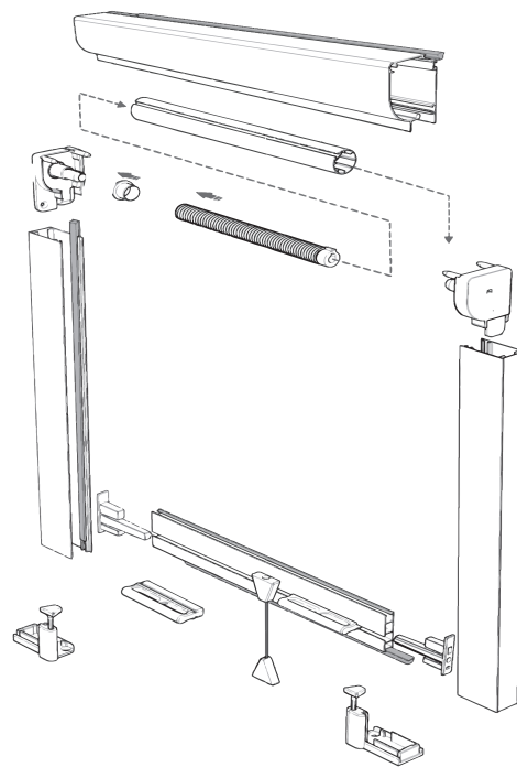
ESQUEMA DE MONTAGEM
