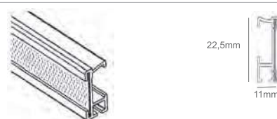
Calha Velcrada Branca
