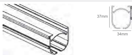
Calha Velcrada Branca Compact Star
